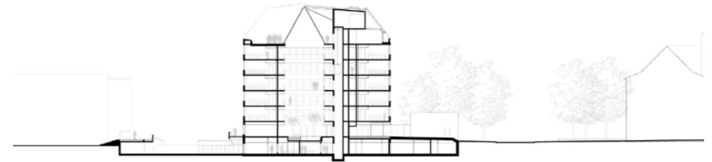
Coupe transversale nord-sud
