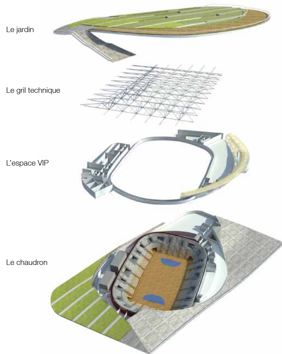
Axonométrie éclatée
